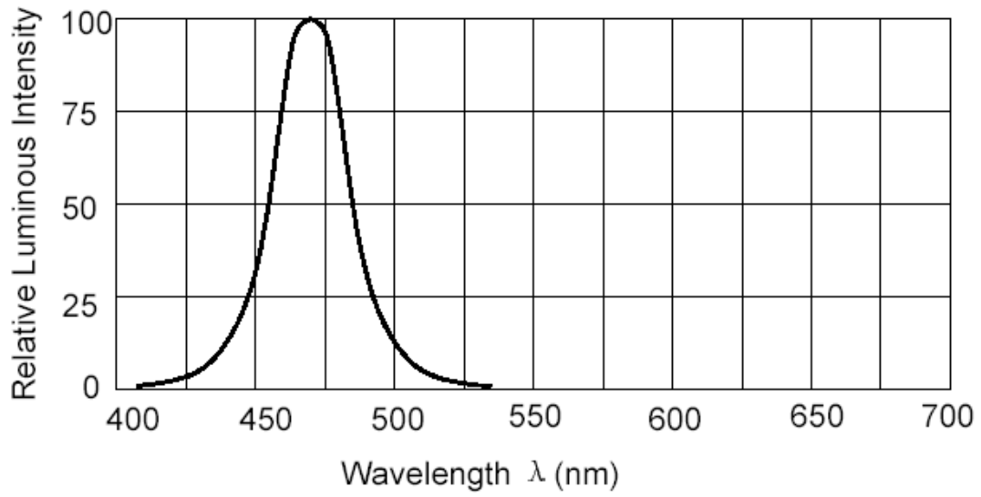
Fig.5 相对亮度 Vs. 波长
