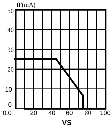
VS AMBIENT TEMPERATURE(Tjmax=105 °C)
