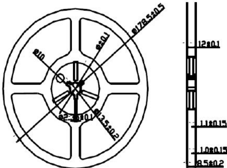
(3) 卷轴尺寸 Reel Dimension
