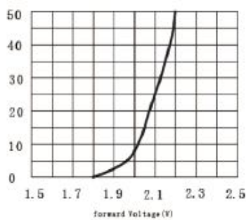
FORWARD CURRENT VS FORWARD VOLTAGE 正向电流和正向电压的关系曲线图
