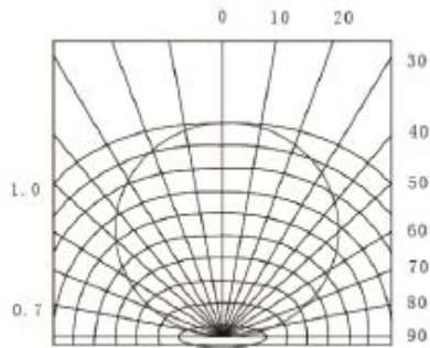
BEAM DISTRIBUTION 发光角度曲线图
