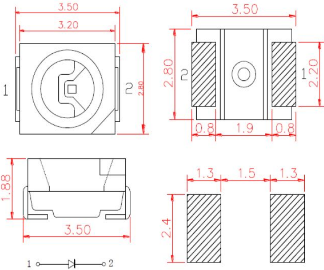
焊盘图
