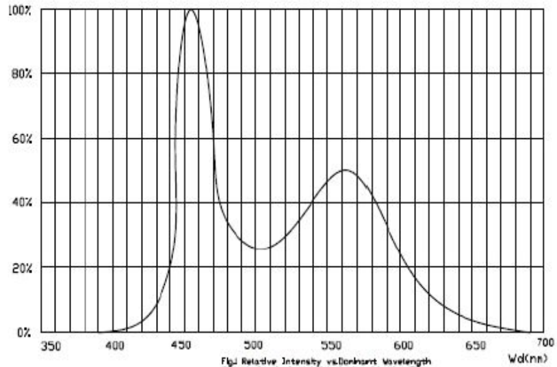
Fig.1 Relative Intensity vs. Wavelength 相对亮度与波长之间的关系
