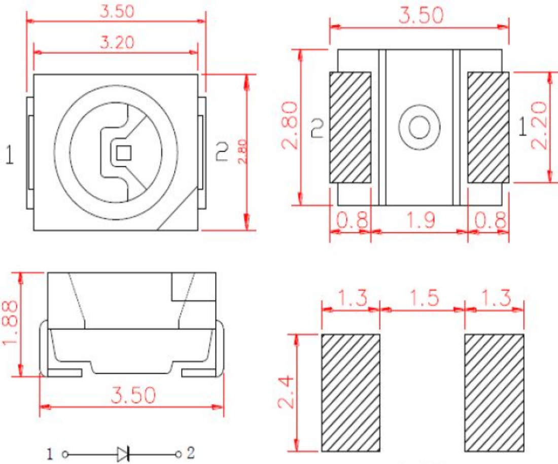
焊盘图
