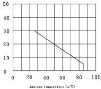
正向电流随温度曲线图
