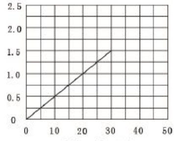
亮度和正向电流关系曲线图
