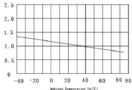
亮度与环境温度关系曲线图
