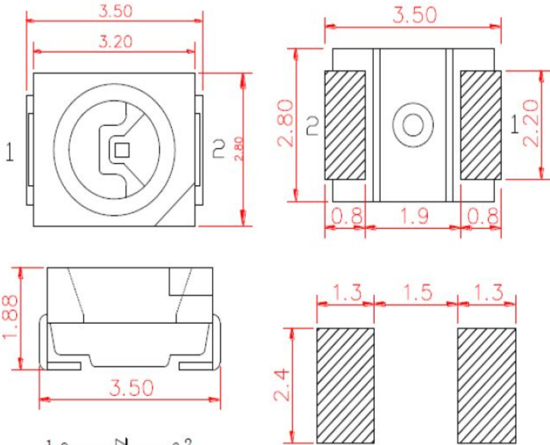
焊盘图
