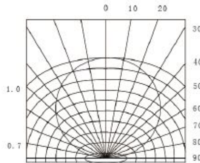
发光角度曲线图
